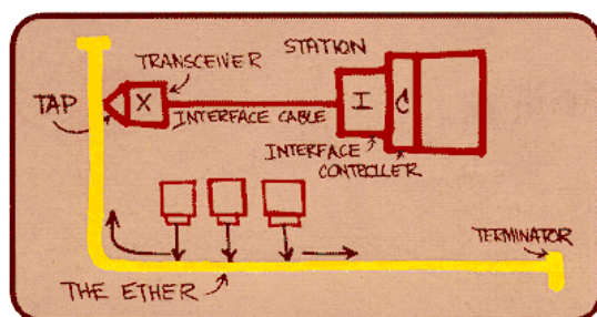
Metcalfe-ova skica Etherneteta
